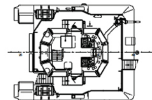
Bridgedeck
